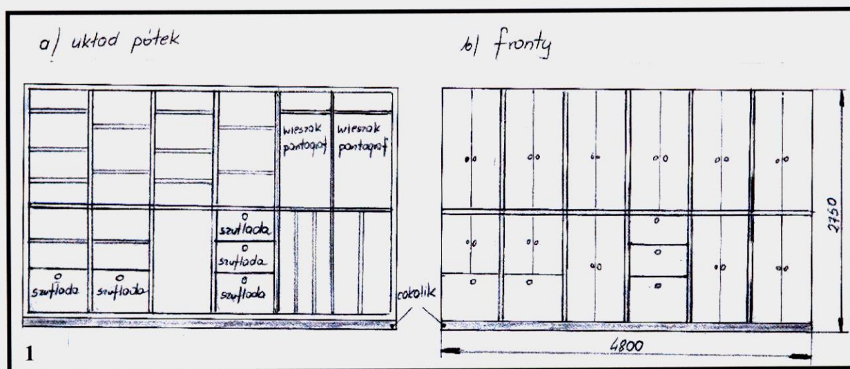
Rysunek Nr 1. Projekt mebli szkolnych
